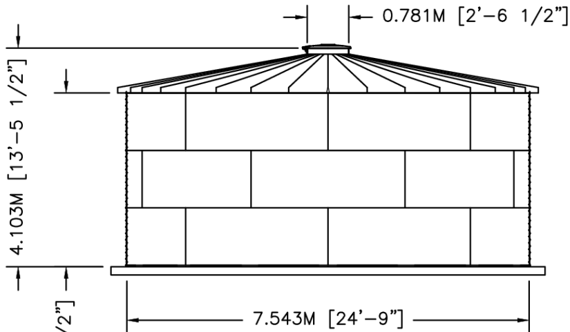
ELEVATION
